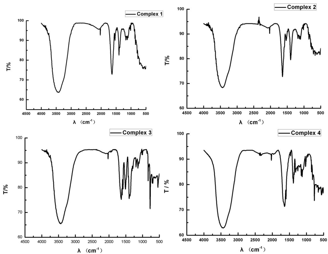
Figure S12. IR Spectra.
