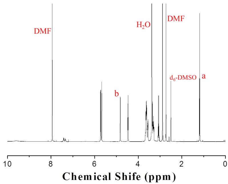
Figure S1 ^1\text{H} NMR spectra of JCD ( 10^{-3} M) ( \text{d}_6\text{-DMSO} ).
