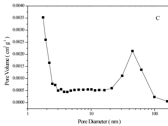
Fig. S3 BET experimental data.
