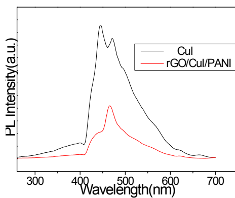
Fig. 3S PL spectra of CuI and rGO/CuI/PANI
