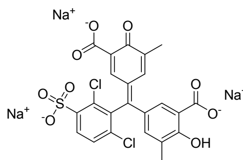
Chrome Azurol S(CAS)
