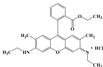
Rhodamine 6G (R6G)
