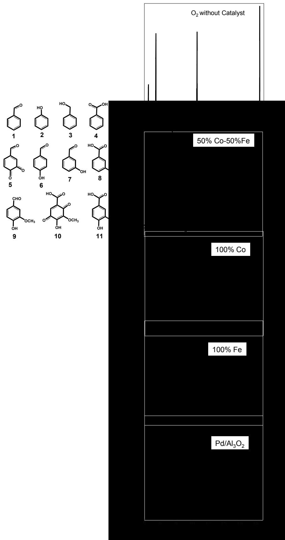
Fig.S2 : GC chromatogrammes of lignin dimer
