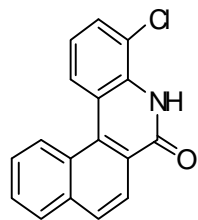
5g DMSO-D6
