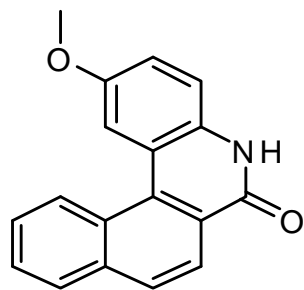
5b DMSO-D6
