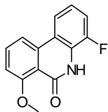
5pl DMSO-D6
