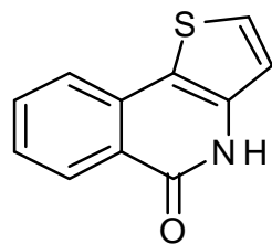
5af DMSO-D6
