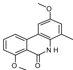
5ec DMSO-D6
