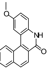
5b
