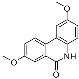
5mb DMSO-D6
