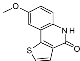
5ob DMSO-D6
