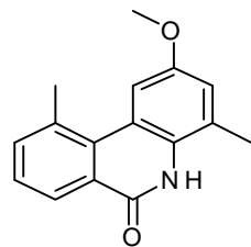
5dc DMSO-D6
