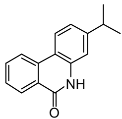
5ae-a DMSO-D6
