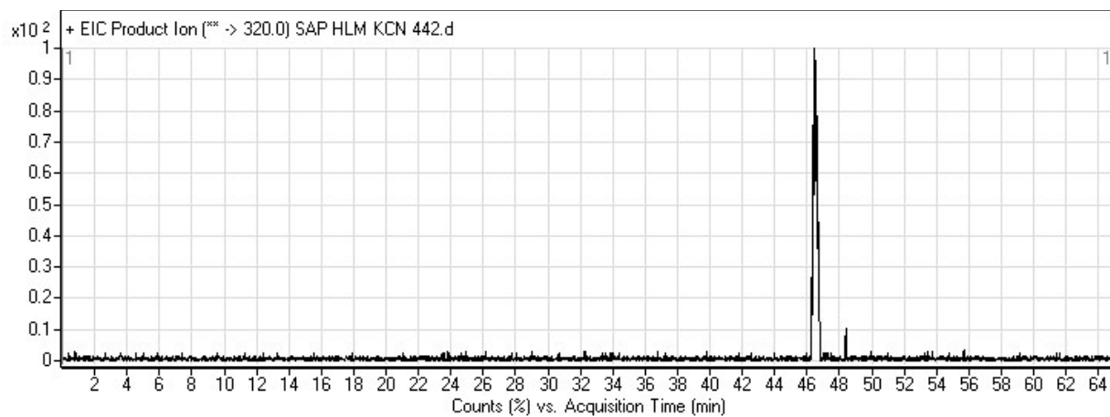
Fig. S7. M8 PI chromatogram.
