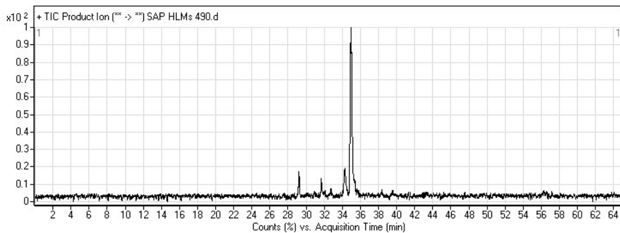
Fig. S5. M4, M5 and M6 PI chromatogram.
