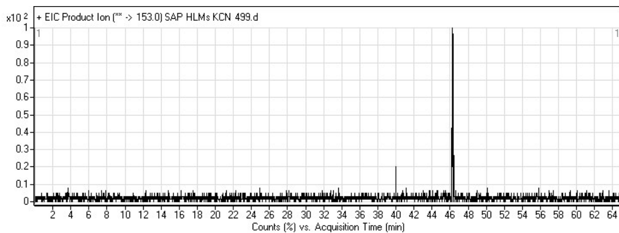
Fig. S6. M7 PI chromatogram.
