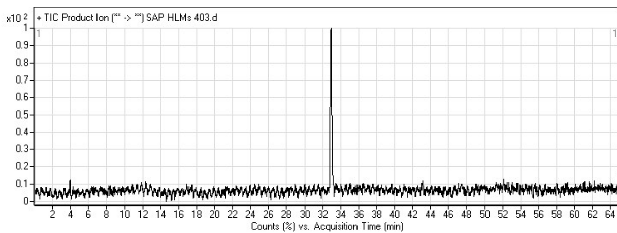
Fig. S4. M3 PI chromatogram.
