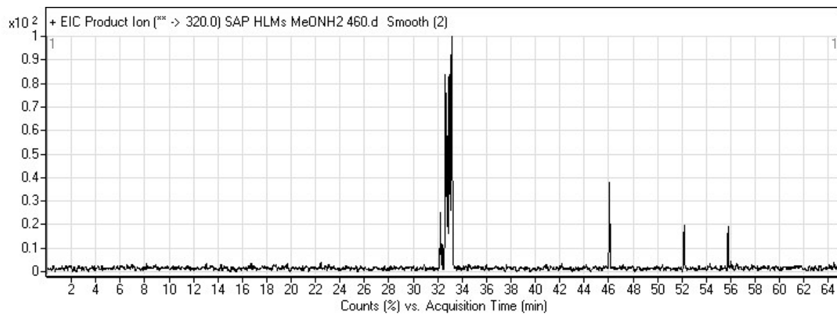
Fig. S8. M9 PI chromatogram.
