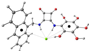
6...Cl -
