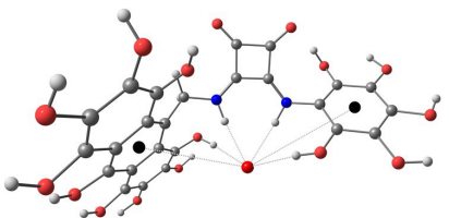
7...Br -
