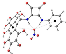
5...NO 3 -
