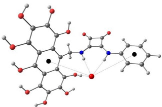
5...Br -
