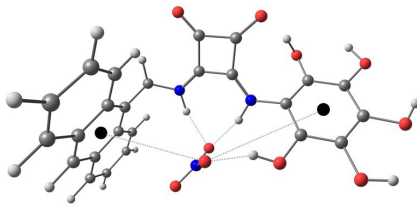
6...NO 3 -
