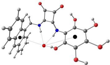
6...Br -
