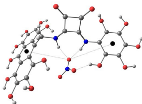
7...NO 3 -
