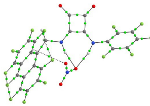
4-NO 3 -
