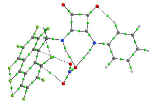
2-NO 3 -
