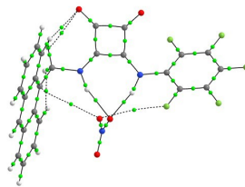
3-NO 3 -
