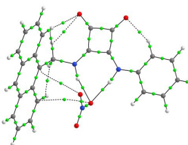
1-NO 3 -
