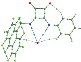
2-Br -
