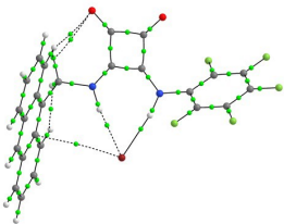
3-Br -
