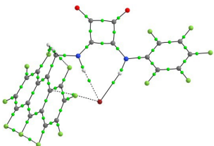
4-Br -
