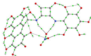
7-NO 3 -
