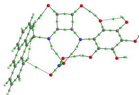
6-NO 3 -
