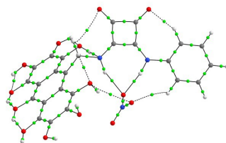
5-NO 3 -
