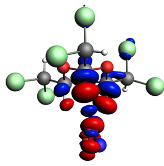
4...NO 2 -*
