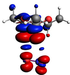
2...NO 2 -1
