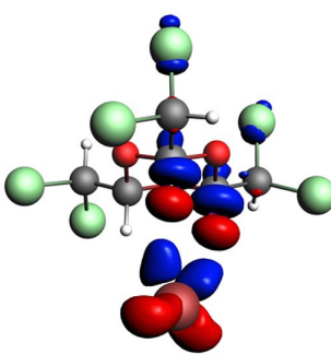
4...Br -*
