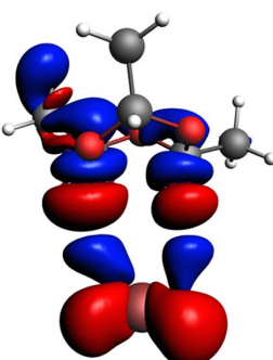
2...Br -e
