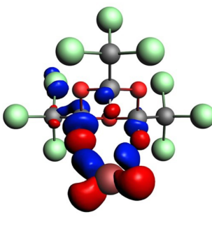
5...Br -*
