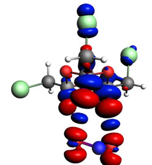
3...NO 2 -phi
