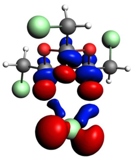
3...Cl -phi
