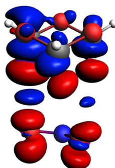
1...NO 2 -1
