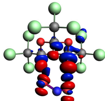
5...NO 2 -*
