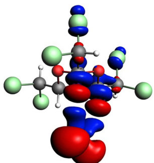
4...Cl -phi
