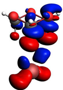
1...Br -1
