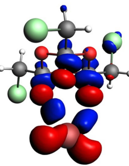
3...Br -phi
