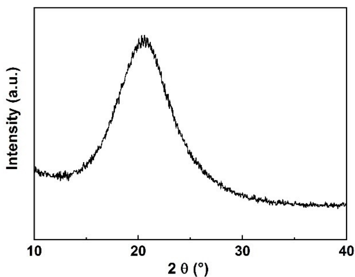
Fig. S1. WAXD of XDI-PUE.
