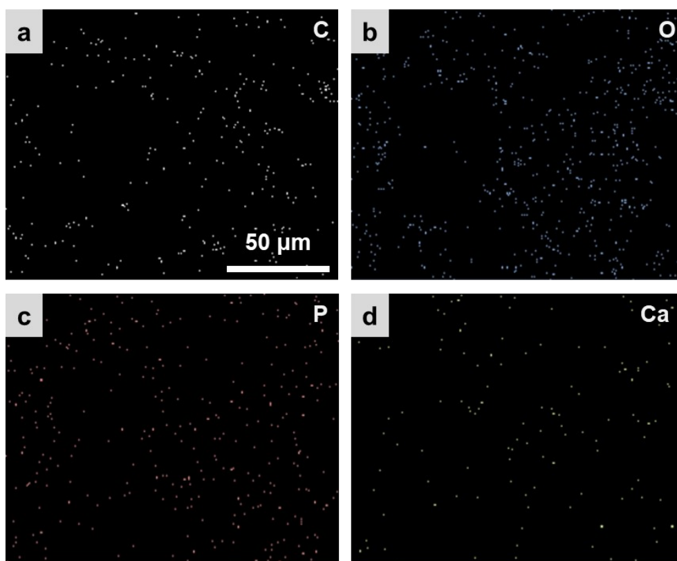
Fig. S1 EDX (a) C, (b) O, (c) P and (d) Ca mapping images of cellulose80_HA2.
