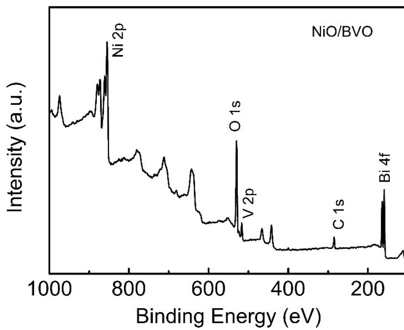
Fig. S2 XPS survey spectrum of NiO/BVO.
