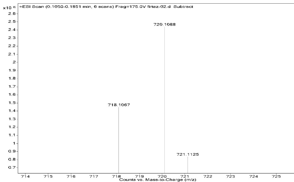
Fig. S6. Mass spectra of IrTAZ.
