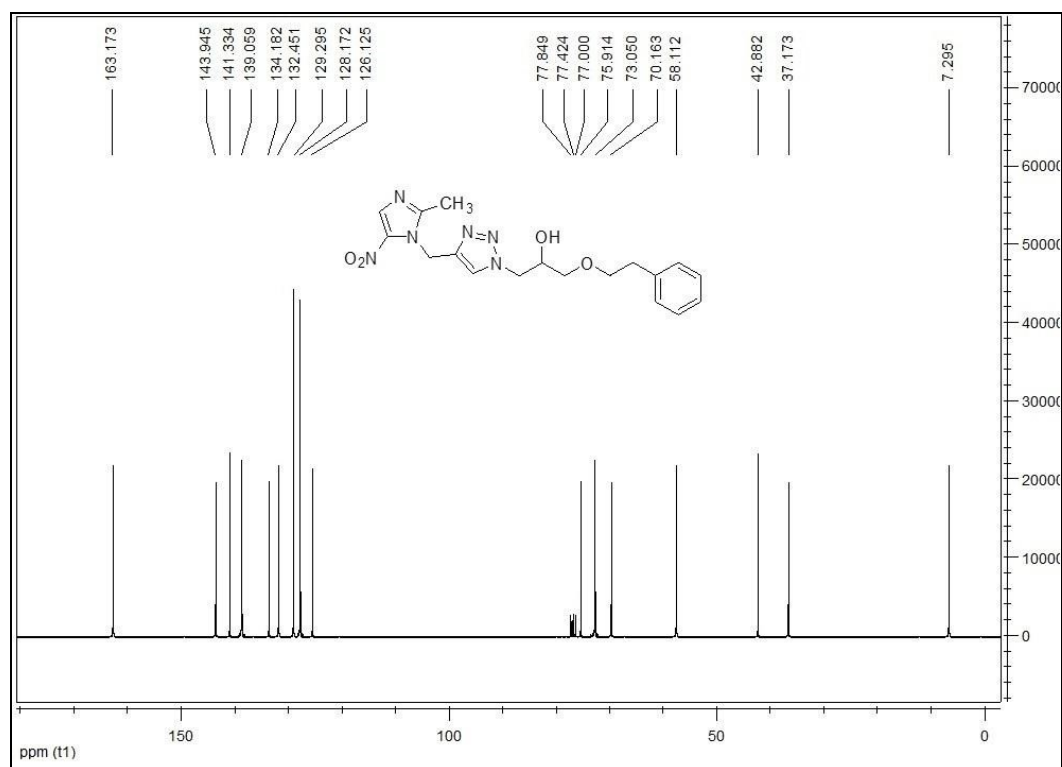
16c: 1-(4-((2-methyl-5-nitro-1H-imidazol-1-yl)methyl)-1H-1,2,3-triazol-1-yl)-3-phenethoxypropan-2-ol
