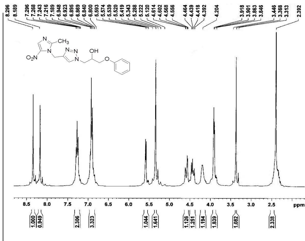
16a: 1-(4-((2-methyl-5-nitro-1H-imidazol-1-yl)methyl)-1H-1,2,3-triazol-1-yl)-3-phenoxypropan-2-ol
