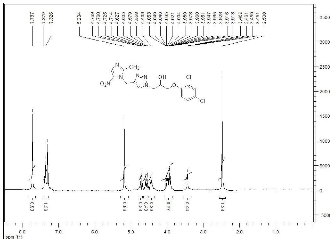
16d: 1-(2,4-dichlorophenoxy)-3-(4-((2-methyl-5-nitro-1H-imidazol-1-yl)methyl)-1H-1,2,3-triazol-1-yl)propan-2-ol
