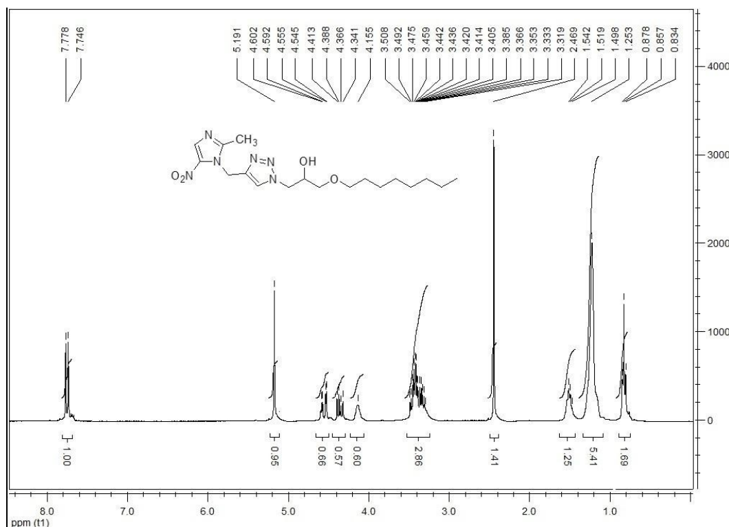
16i: 1-(4-((2-methyl-5-nitro-1H-imidazol-1-yl)methyl)-1H-1,2,3-triazol-1-yl)-3-(octyloxy)propan-2-ol
