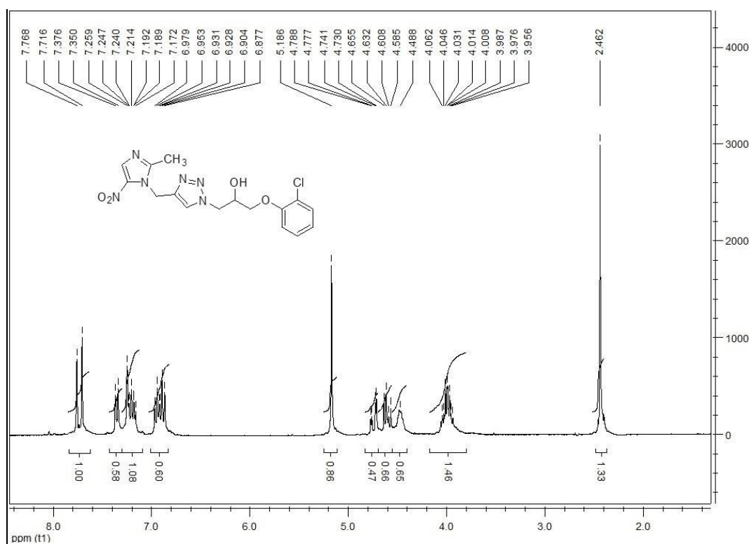
16e: 1-(2-chlorophenoxy)-3-(4-((2-methyl-5-nitro-1H-imidazol-1-yl)methyl)-1H-1,2,3-triazol-1-yl)propan-2-ol
