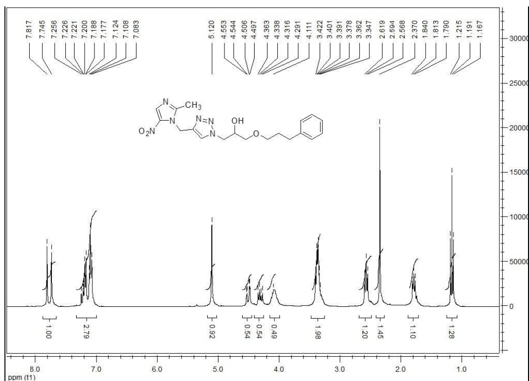
16j : 1-(4-((2-methyl-5-nitro-1H-imidazol-1-yl)methyl)-1H-1,2,3-triazol-1-yl)-3-(3-phenylpropoxy)propan-2-ol
