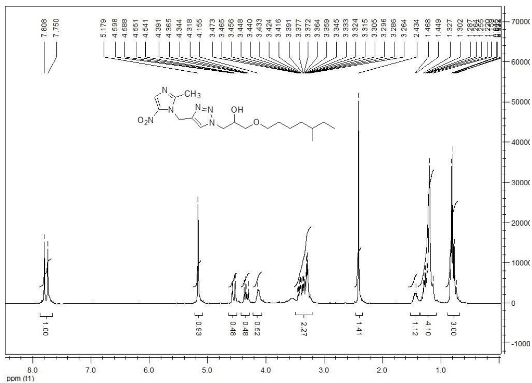
16h: 1-(4-((2-methyl-5-nitro-1H-imidazol-1-yl)methyl)-1H-1,2,3-triazol-1-yl)-3-((5-methylheptyl)oxy)propan-2-ol
