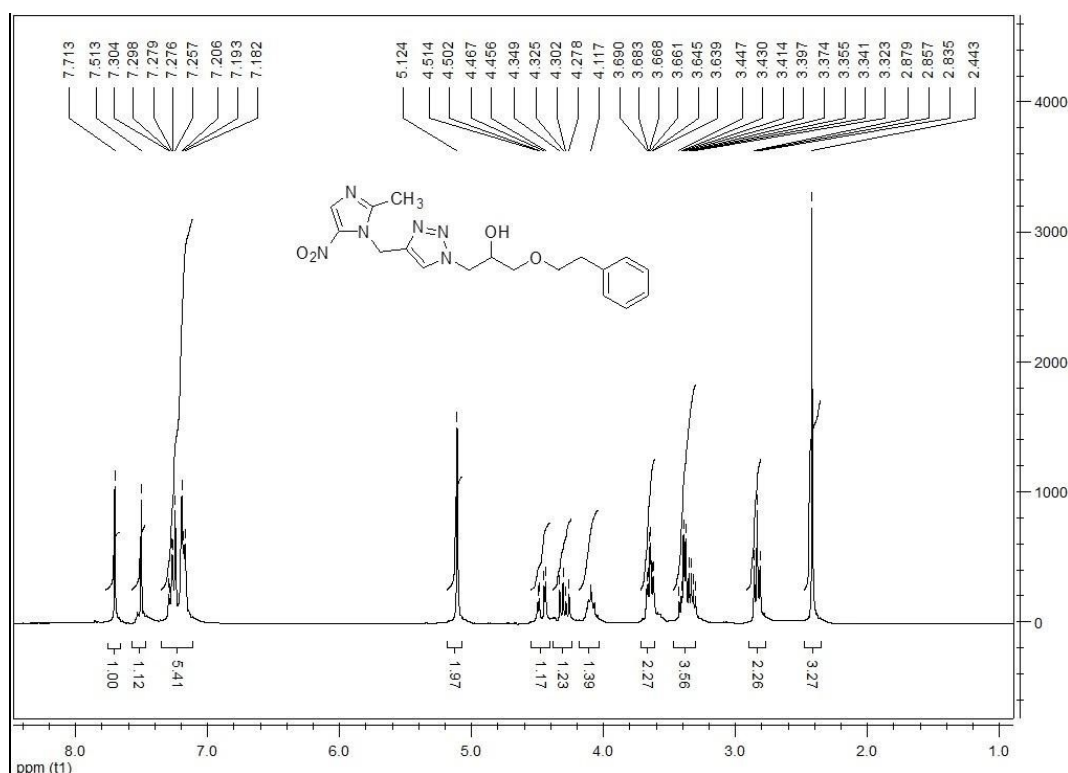
16c: 1-(4-((2-methyl-5-nitro-1H-imidazol-1-yl)methyl)-1H-1,2,3-triazol-1-yl)-3-phenethoxypropan-2-ol
