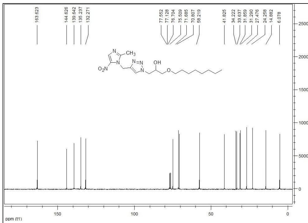
16i: 1-(4-((2-methyl-5-nitro-1H-imidazol-1-yl)methyl)-1H-1,2,3-triazol-1-yl)-3-(octyloxy)propan-2-ol
