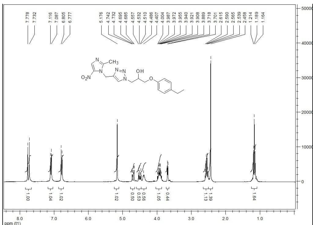
16g: 1-(4-ethylphenoxy)-3-(4-((2-methyl-5-nitro-1H-imidazol-1-yl)methyl)-1H-1,2,3-triazol-1-yl)propan-2-ol
