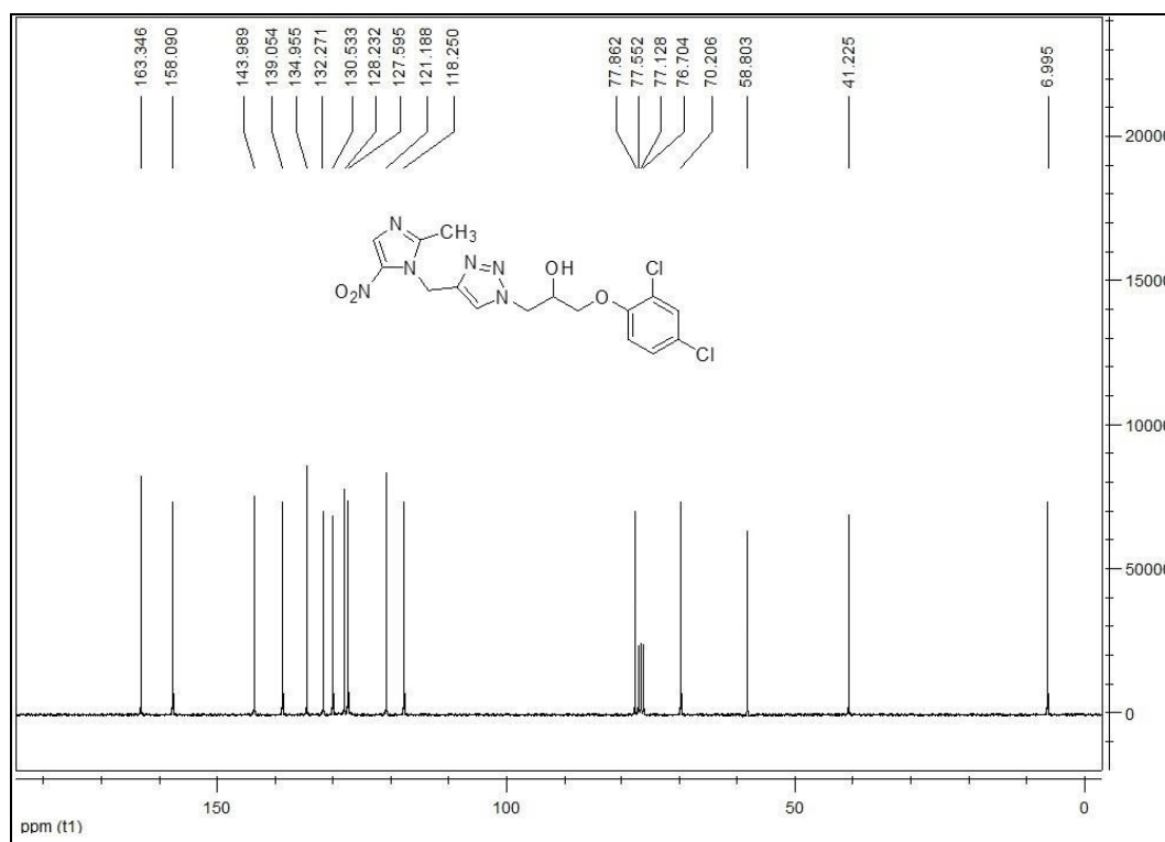
16d: 1-(2,4-dichlorophenoxy)-3-(4-((2-methyl-5-nitro-1H-imidazol-1-yl)methyl)-1H-1,2,3-triazol-1-yl)propan-2-ol
