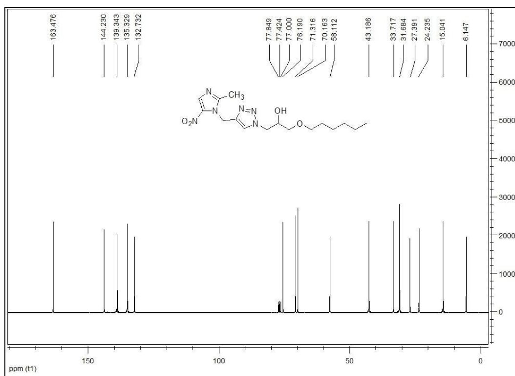
16k: 1-(hexyloxy)-3-(4-((2-methyl-5-nitro-1H-imidazol-1-yl)methyl)-1H-1,2,3-triazol-1-yl)propan-2-ol
