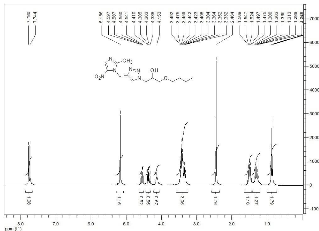
16b: 1-butoxy-3-(4-((2-methyl-5-nitro-1H-imidazol-1-yl)methyl)-1H-1,2,3-triazol-1-yl)propan-2-ol
