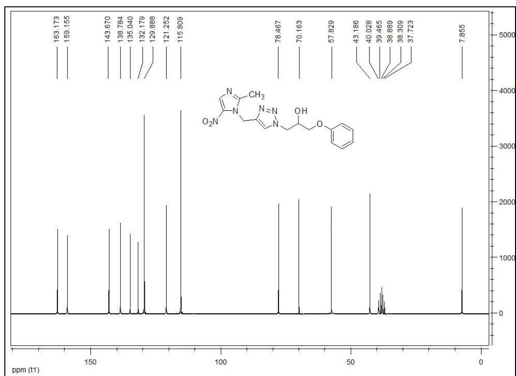
16a: 1-(4-((2-methyl-5-nitro-1H-imidazol-1-yl)methyl)-1H-1,2,3-triazol-1-yl)-3-phenoxypropan-2-ol
