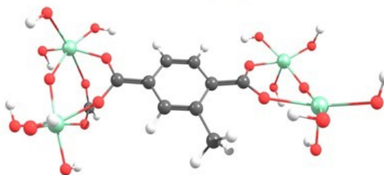
M-CH 3 /S 1
