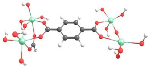
M-(vac)/T 1
