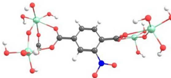
M-NO 2 /T 1
