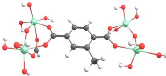
M-CH 3 /T 1
