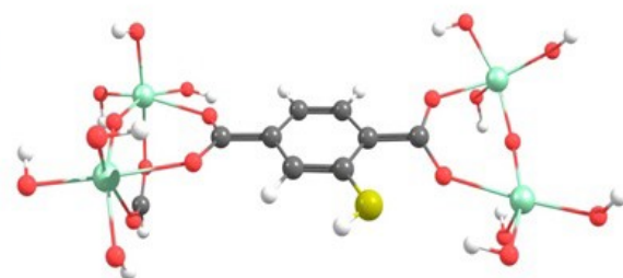
M-SH/T 1
