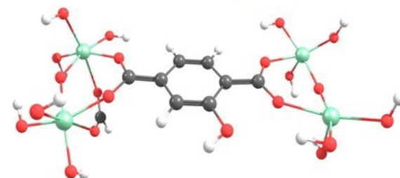
M-OH/S 1
