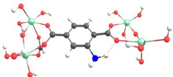
M-NH 2 /S 1
