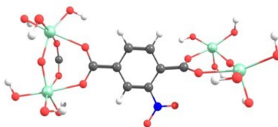
M-NO 2 /S 1
