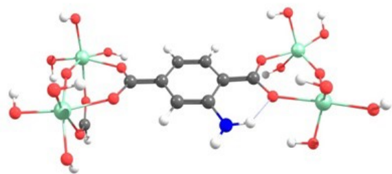
M-NH 2 /T 1
