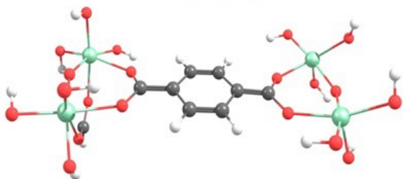
M-(vac)/S 1
