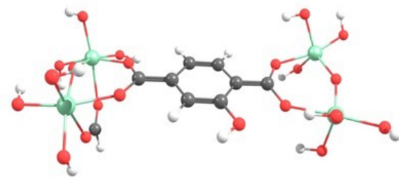
M-OH/T 1
