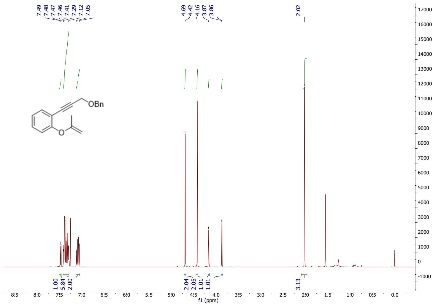
1n: 1-(3-(benzyloxy)prop-1-yn-1-yl)-2-(prop-1-en-2-yloxy)benzene
