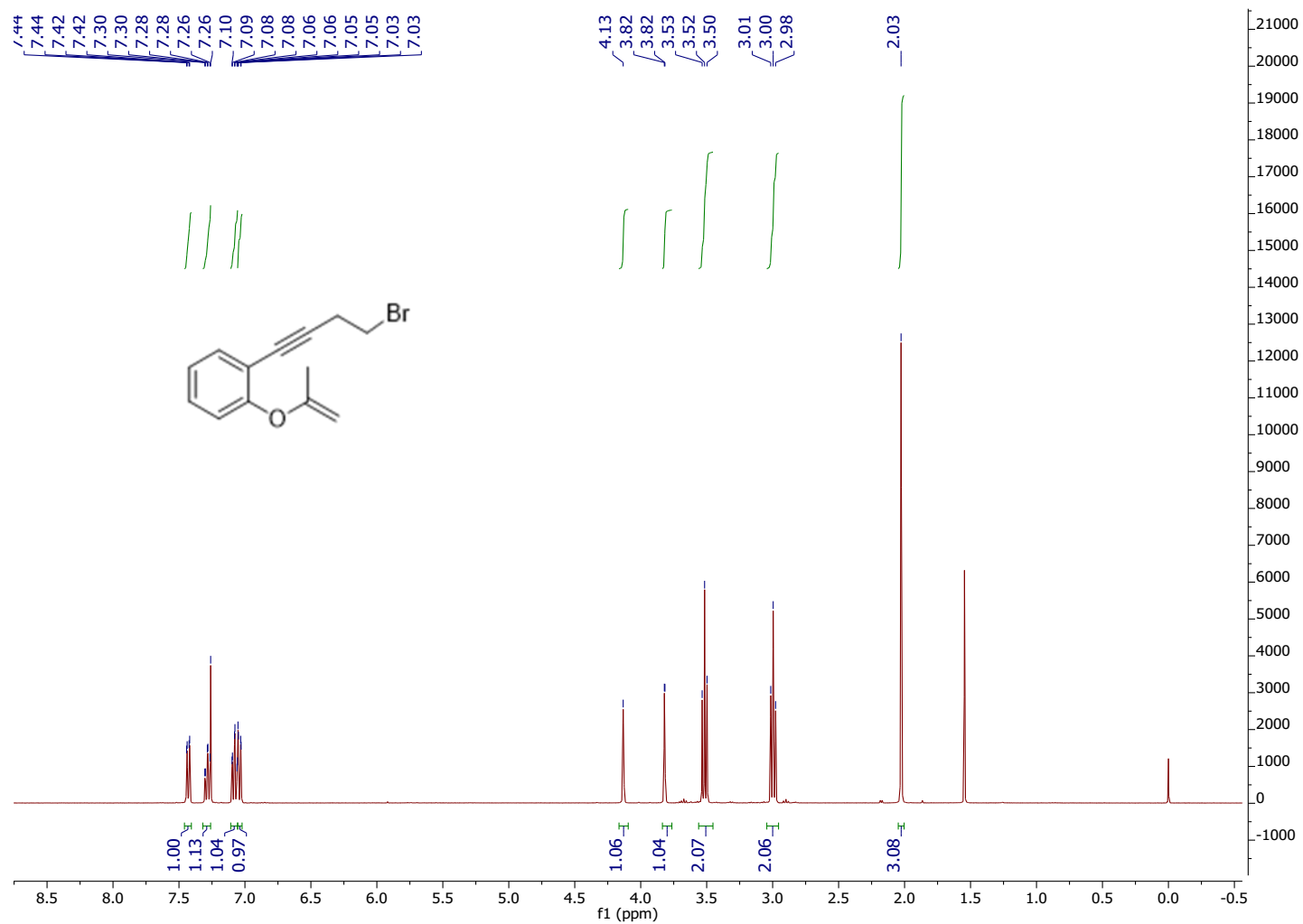
1r: 1-(4-bromobut-1-yn-1-yl)-2-(prop-1-en-2-yloxy)benzene
