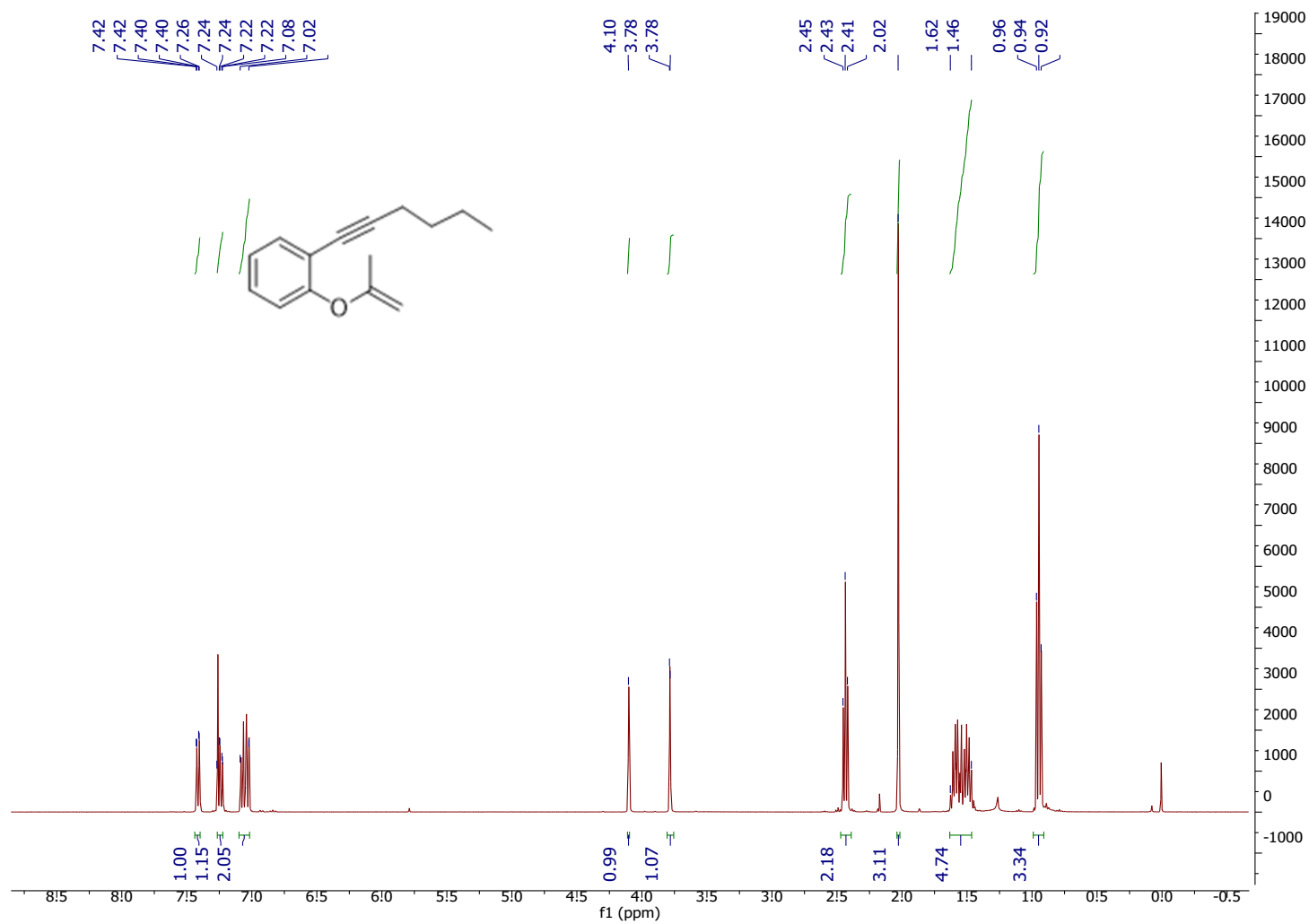
1o: 1-(hex-1-yn-1-yl)-2-(prop-1-en-2-yloxy)benzene
