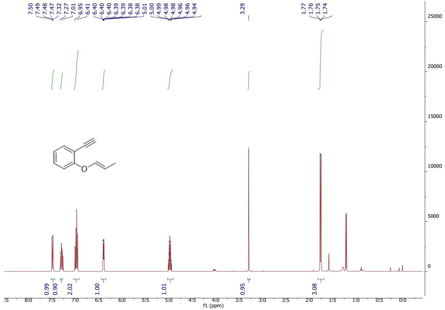
1i: (E)-1-ethynyl-2-(prop-1-en-1-yloxy)benzene
