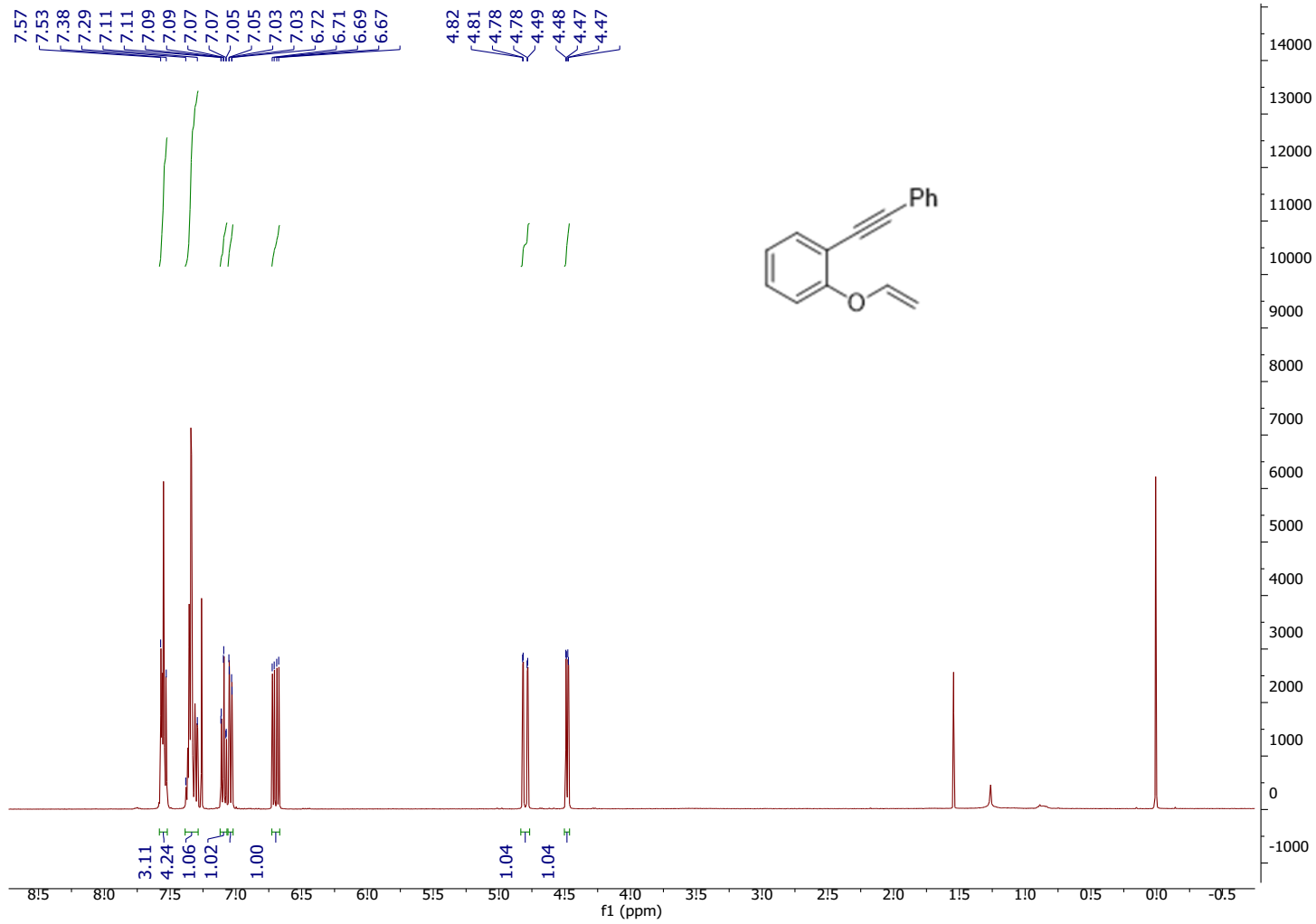
1g: 1-(phenylethynyl)-2-(vinylloxy)benzene
