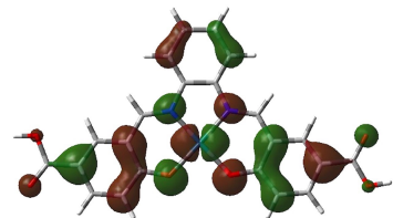
HOMO
