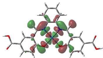
LUMO+4
