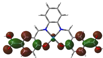
LUMO+2
