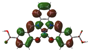
LUMO+1
