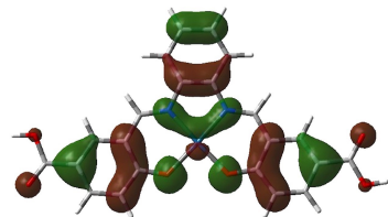
HOMO-1
