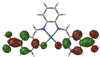
LUMO+3
