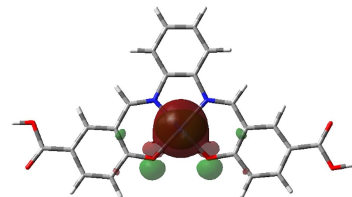
HOMO-3
