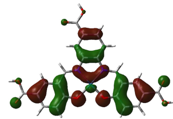
HOMO-1
