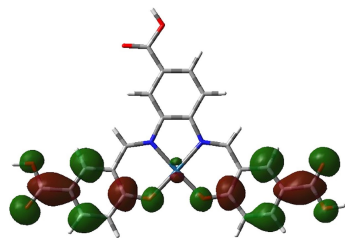
LUMO+3
