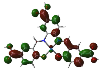
LUMO+2
