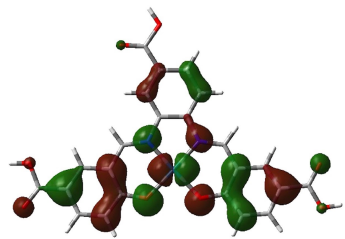
HOMO
