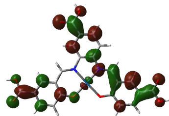
LUMO+4
