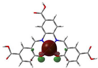
HOMO-3
