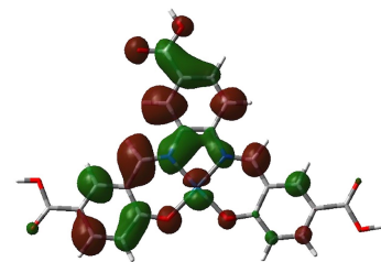
LUMO+1
