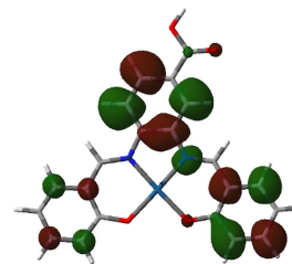
LUMO+4
