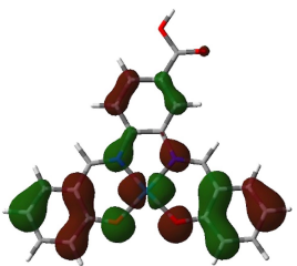
HOMO
