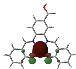
HOMO-3
