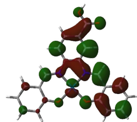
LUMO+1
