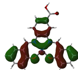
HOMO-1
