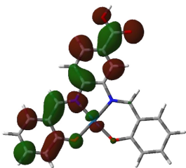
LUMO+2
