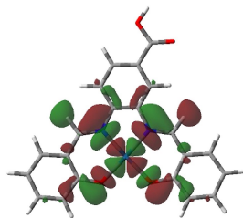
LUMO+3
