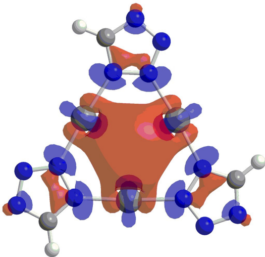
1 , LUMO
