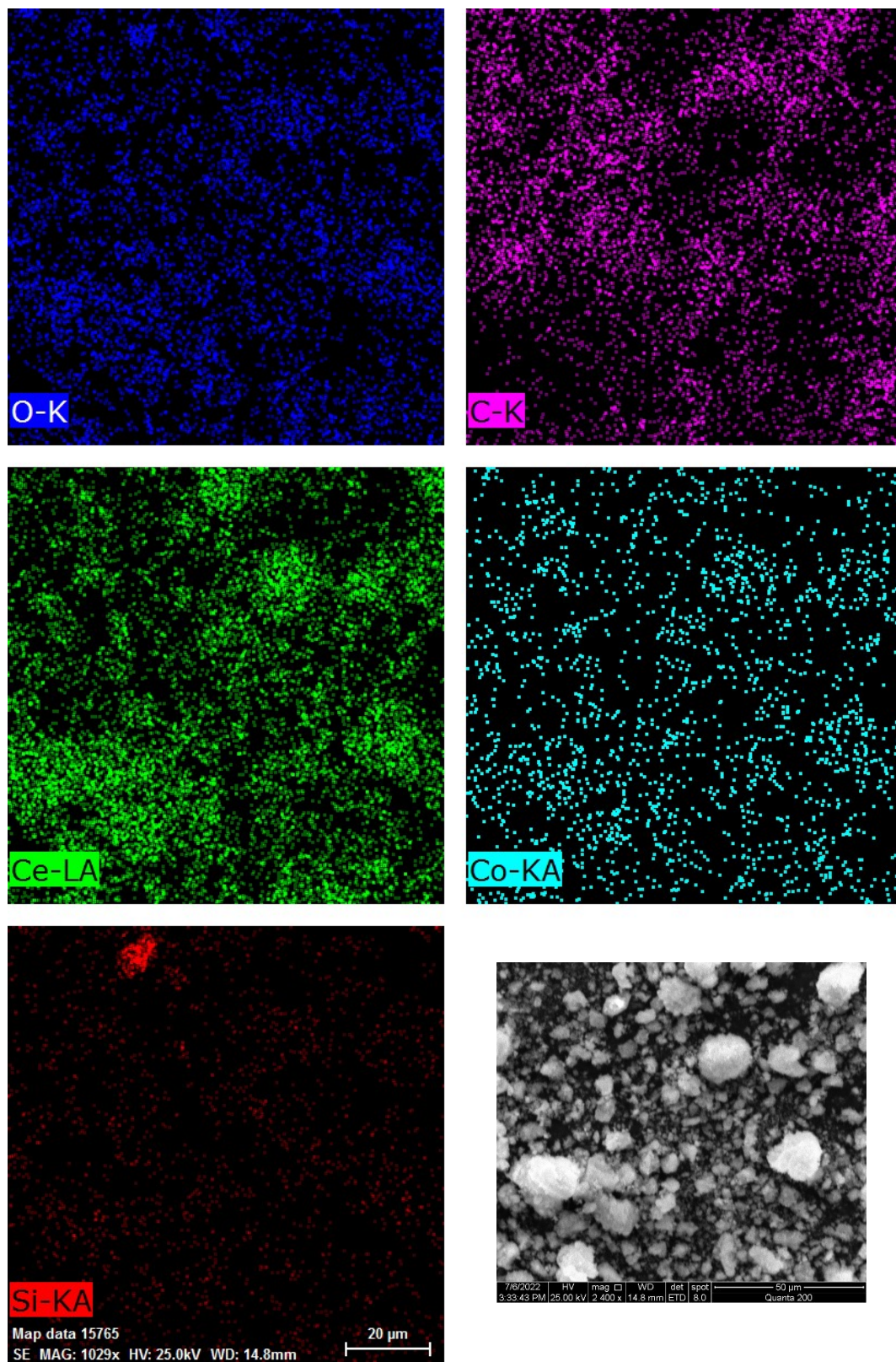
Fig. S1. FESEM/Map data of NC-V Catalyst.
