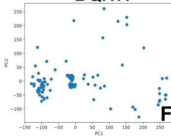
BQ.1.1
