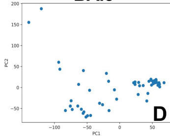
BA.3
