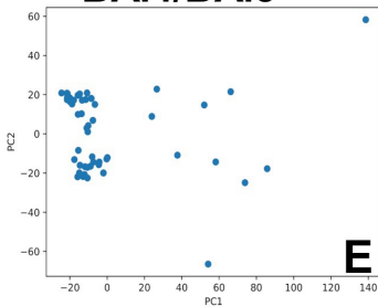
BA.4/BA.5
