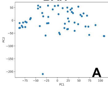
BA.3
