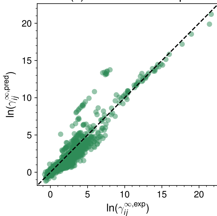
(d) COSMO-SAC-dsp
