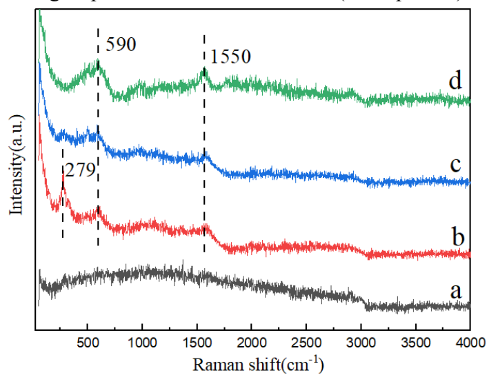
Fig.2s Raman spectra of catalysts (a) 30Cu/SiO 2 ; (b) 30Cu 2 Bi/SiO 2 ; (c) 30Cu 2 Mg/SiO 2 ; (d) 30Cu 2 Mn/SiO 2 ;
