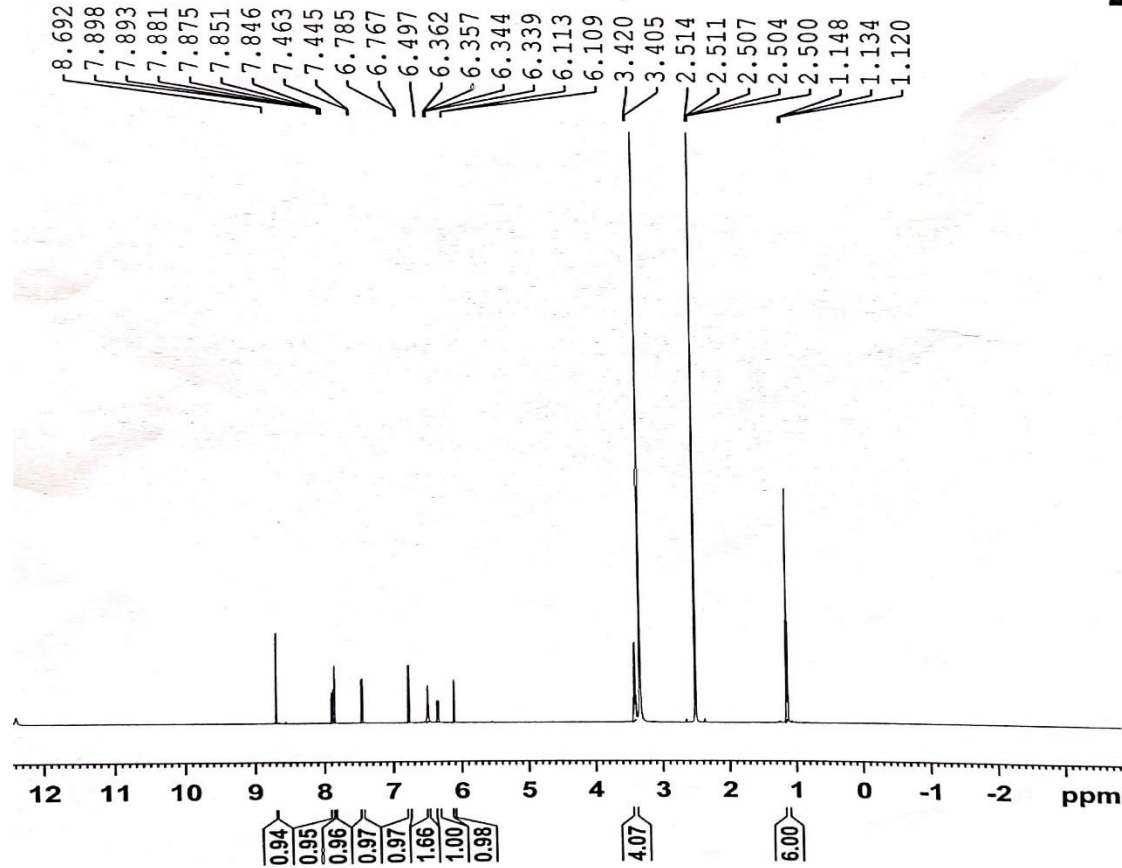
1 H-NMR spectrum of HSB-1
