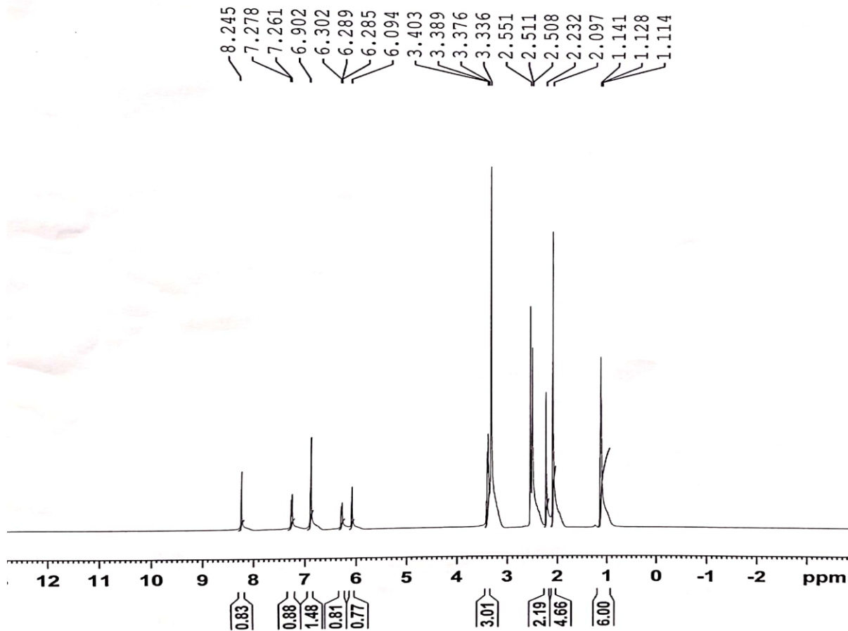
1 H-NMR spectrum of HSB-2
