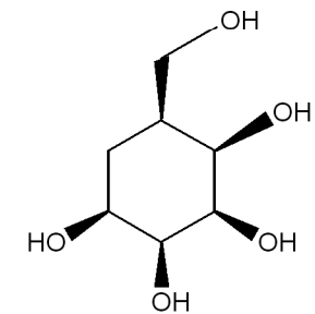
18 Carba-β-L-talopyranose
