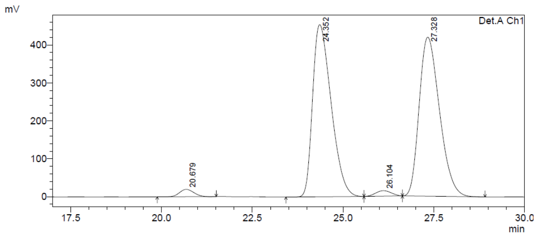
1 Det.A Ch1/254nm
