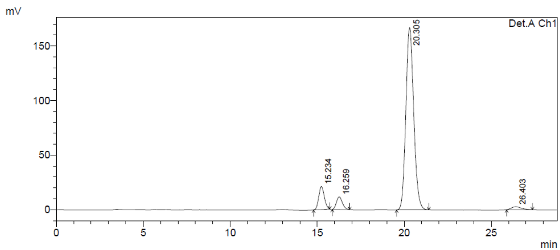
1 Det.A Ch1/254nm
