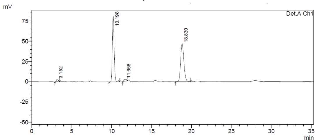
1 Det.A Ch1/254nm
