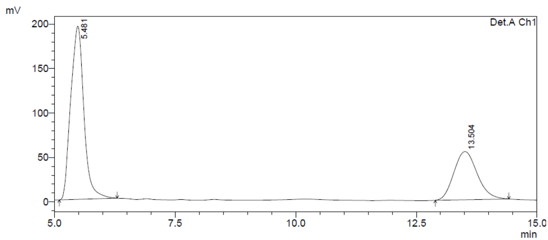
1 Det.A Ch1/254nm
