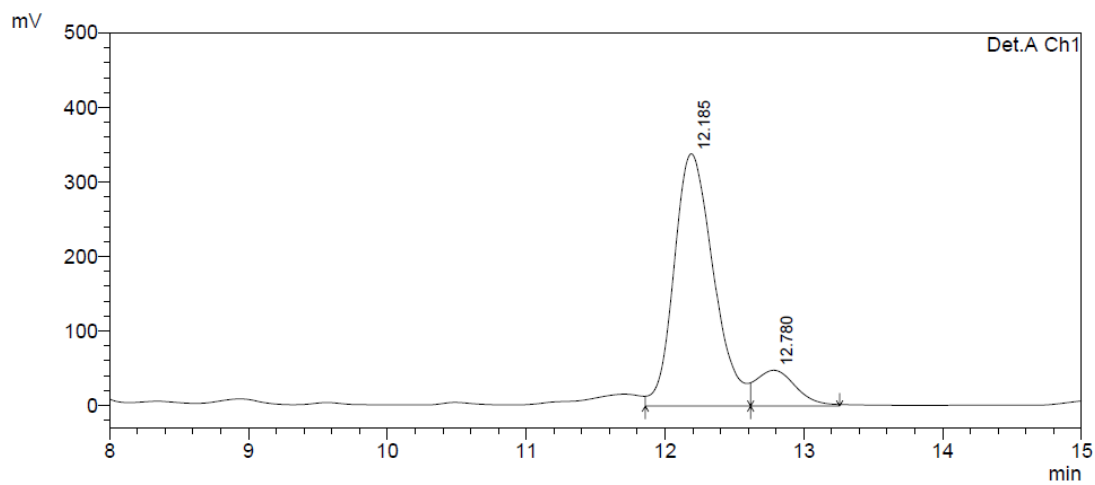
1 Det.A Ch1/254nm
