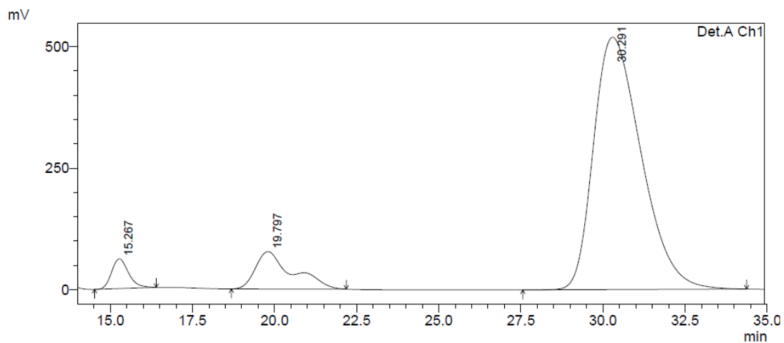
1 Det.A Ch1/254nm
