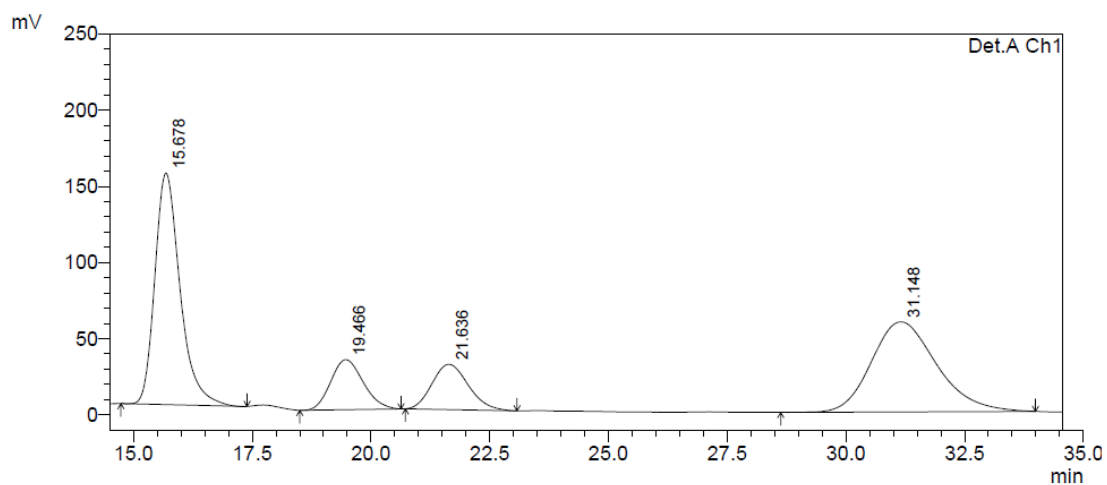
1 Det.A Ch1/254nm
