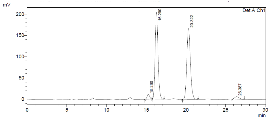
1 Det.A Ch1/254nm
