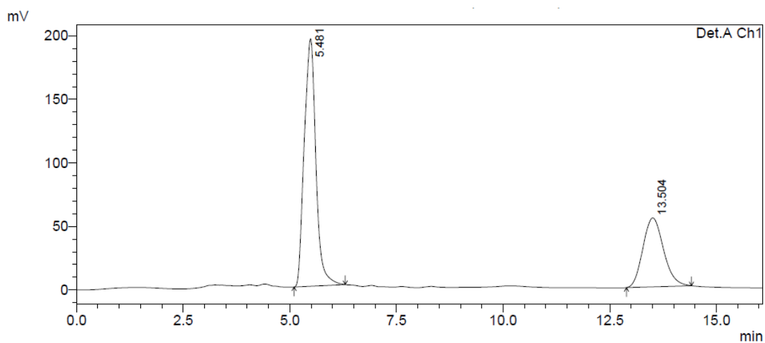
1 Det.A Ch1/254nm
