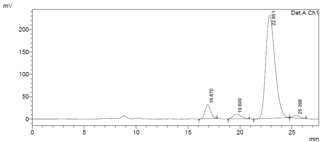
1 Det.A Ch1/254nm
