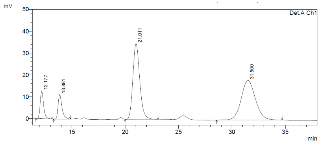
1 Det.A Ch1/254nm
