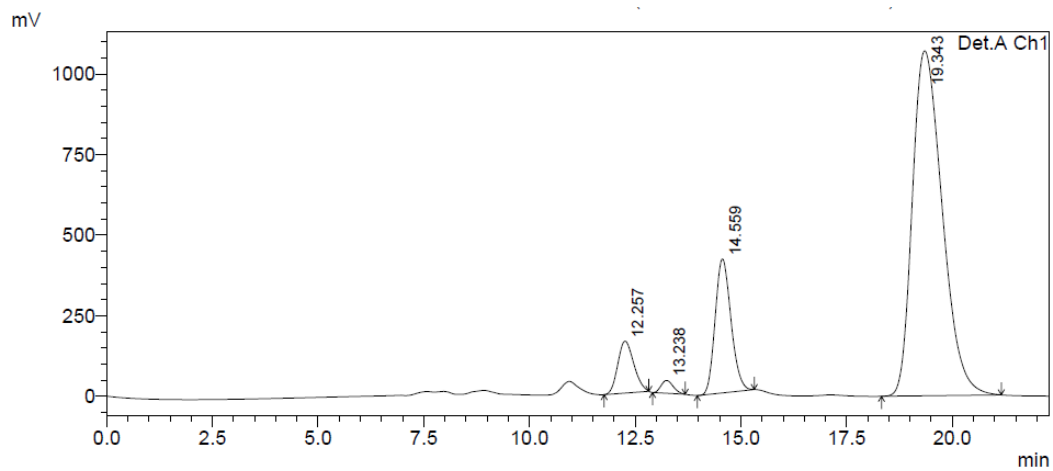
1 Det.A Ch1/254nm
