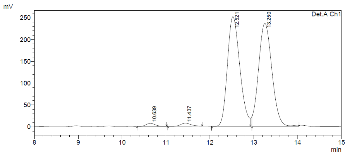
1 Det.A Ch1/254nm
