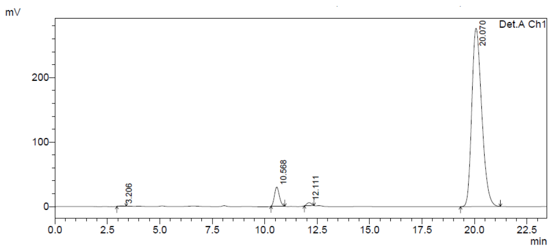
1 Det.A Ch1/254nm
