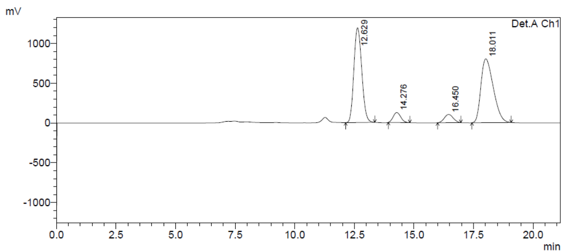
1 Det.A Ch1/254nm
