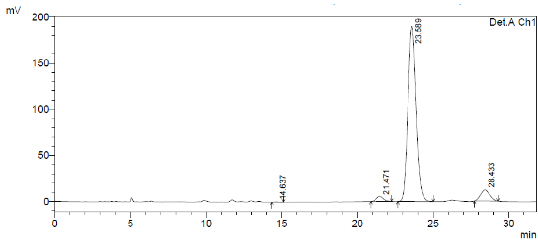
1 Det.A Ch1/254nm
