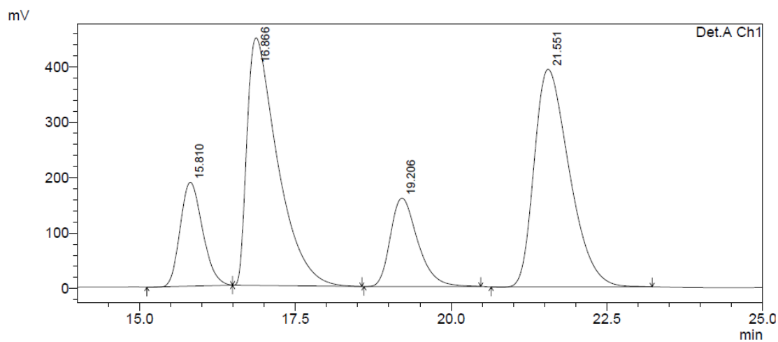
1 Det.A Ch1/254nm
