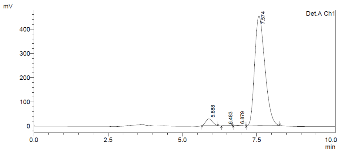
1 Det.A Ch1/254nm
