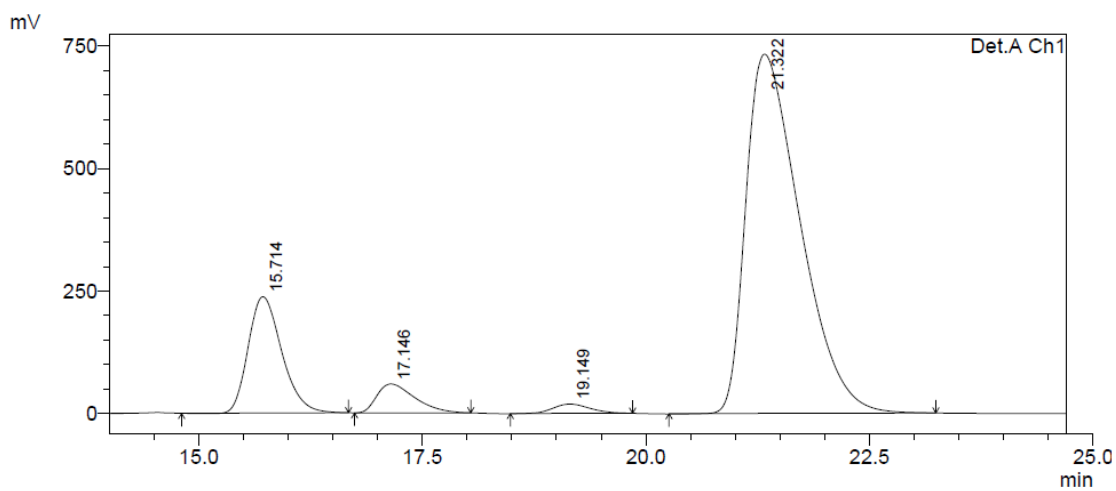
1 Det.A Ch1/254nm
