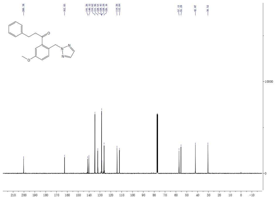
1 H-4f
