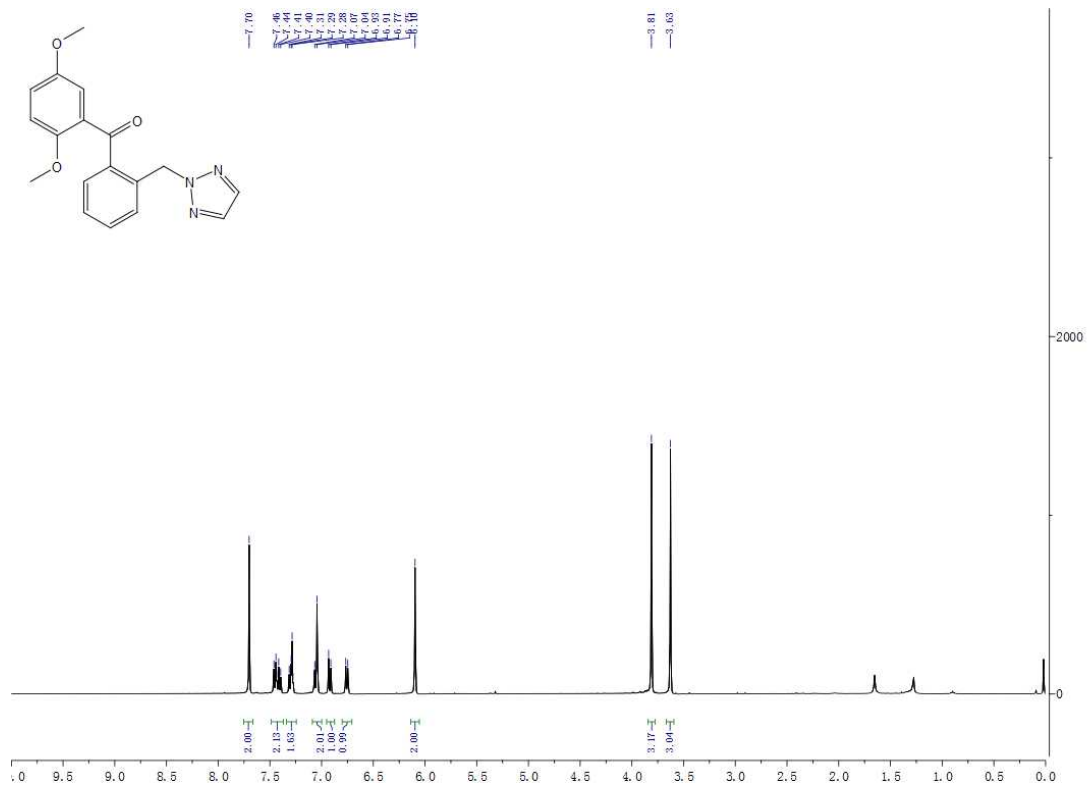
1H-3c
