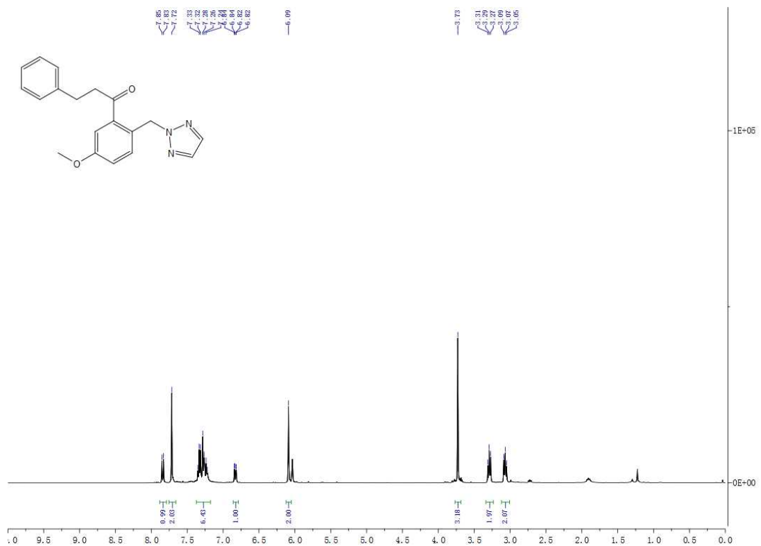
13 C-4e
