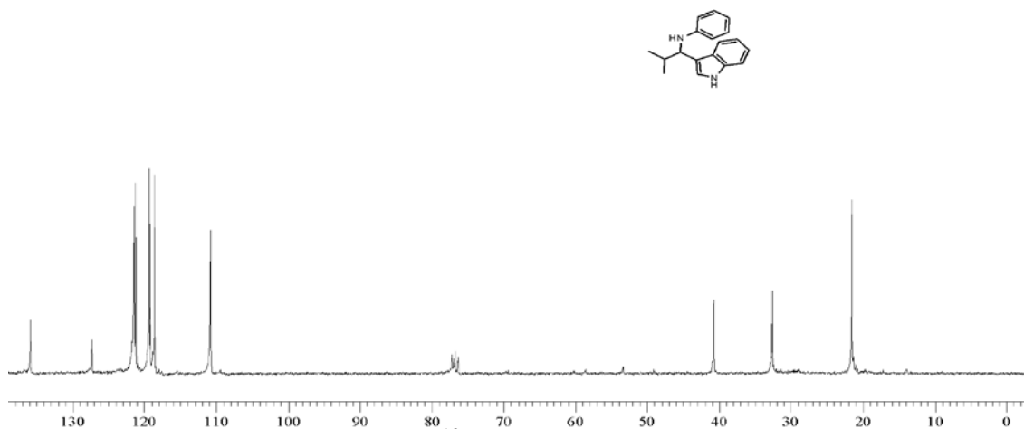
Fig. 38 13 C NMR of compound 4E
