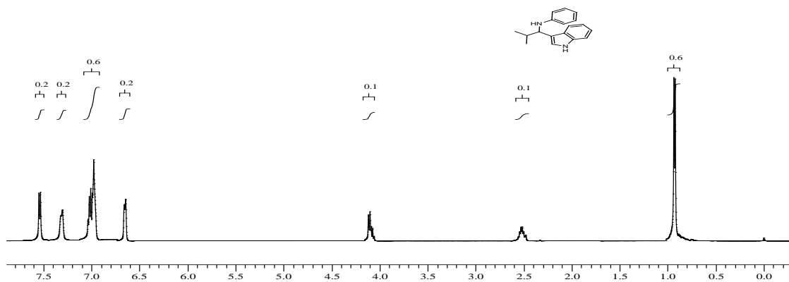
Fig. 37 1 H NMR of compound 4E
