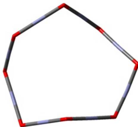
Zn 8 O 8
