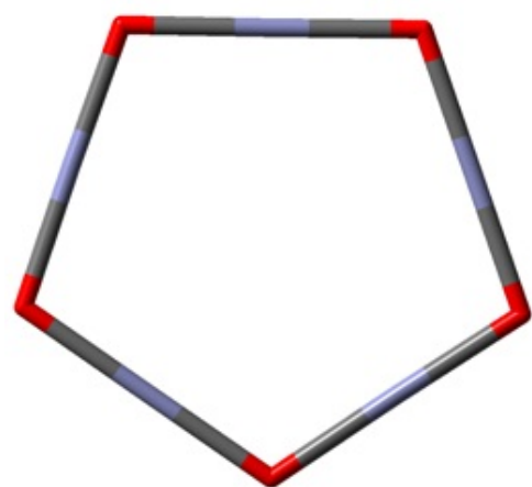
Zn 5 O 5
