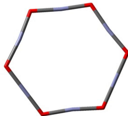
Zn 6 O 6
