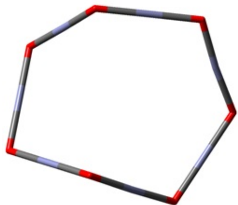
Zn 7 O 7
