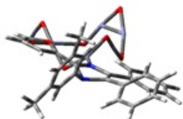
Imidazole-Zn 7 O 7
