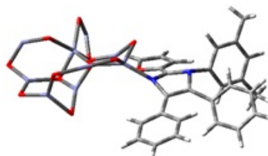
Imidazole-Zn 10 O 10
