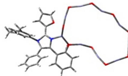
Imidazole-Zn 9 O 9
